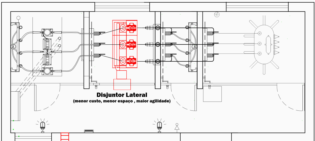
Disjuntor Lateral
