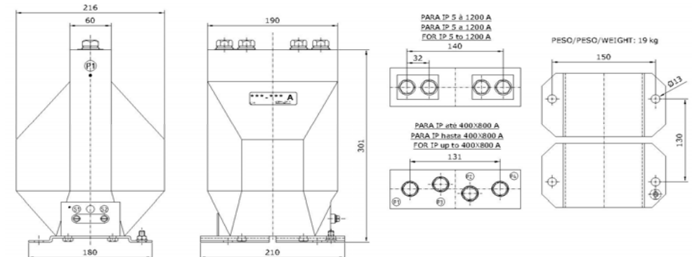
DIMENSÕES / DIMENSIONES / DIMENSIONS(mm)
