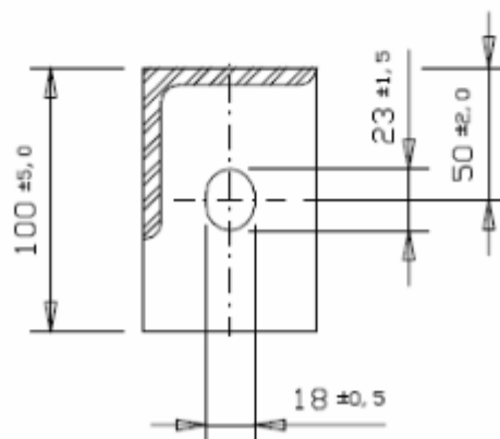
CORTE F-F'
