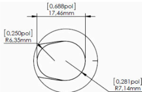
DETALHE B ESCALA 1 : 1
