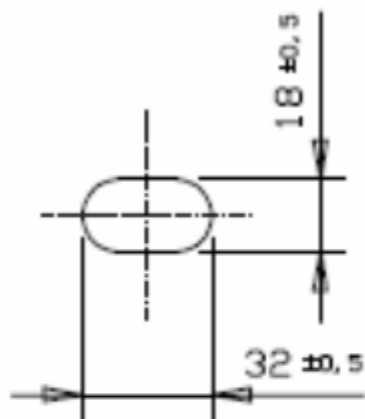
DETALHE DO FURO
