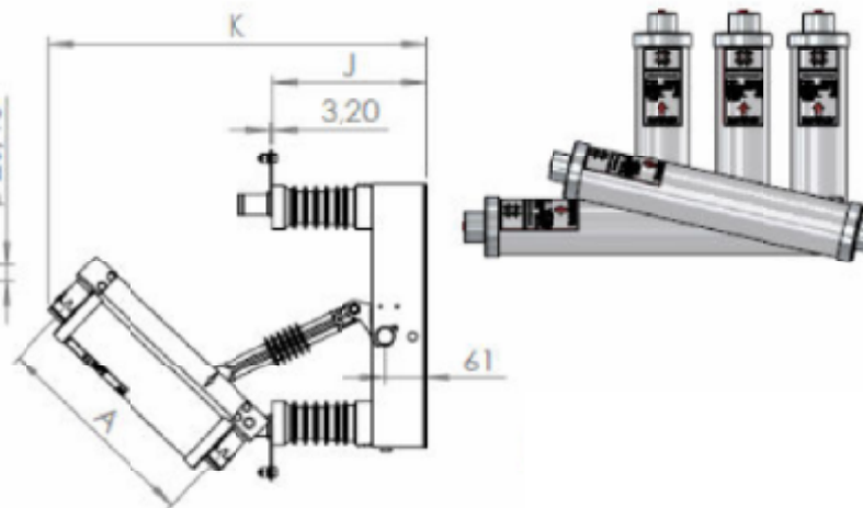
Fusível Limitador de Corrente tipo HH (Veja modelos e detalhes no catálogo)
