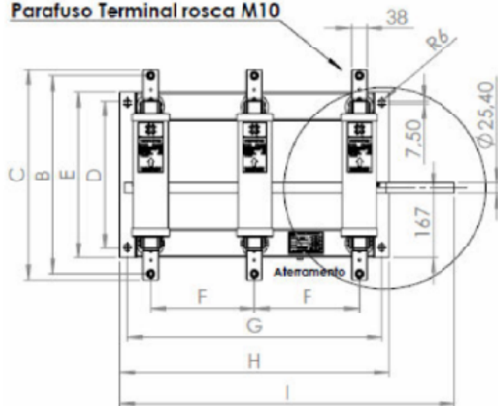
Parafuso Terminal rosca M10
