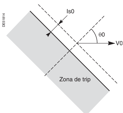
Característica de trip da proteção ANSI 67N/67NC tipo 1 (ângulo característico \theta \neq 0^\circ ).
