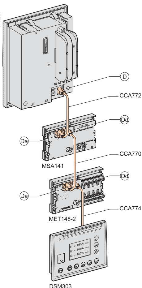
Exemplo de ligação dos módulos para Sepam série 20.
