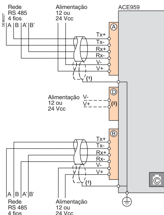
(1) Alimentação remota na fiação separada ou incluída no cabo blindado (3 pares). (2) Borneira para conexão do módulo que fornece a alimentação remota.
