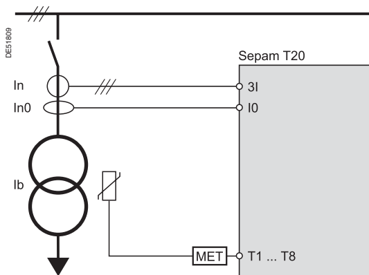
Entradas dos sensores do Sepam T20.
